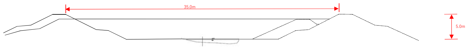
決壊箇所付近横断面図
